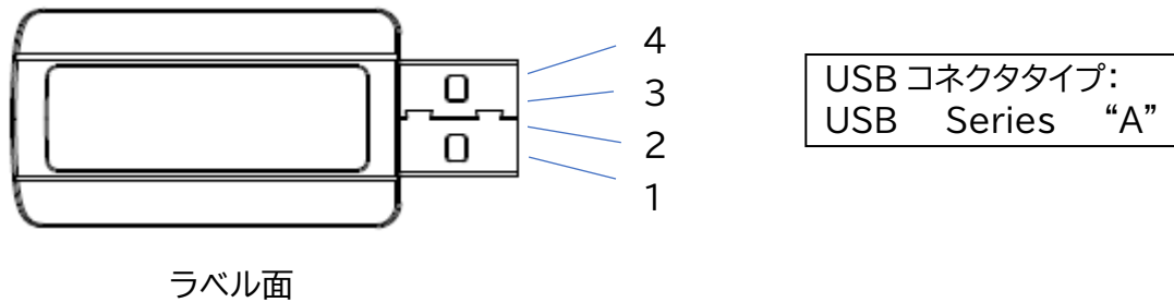
図 2 端子位置
